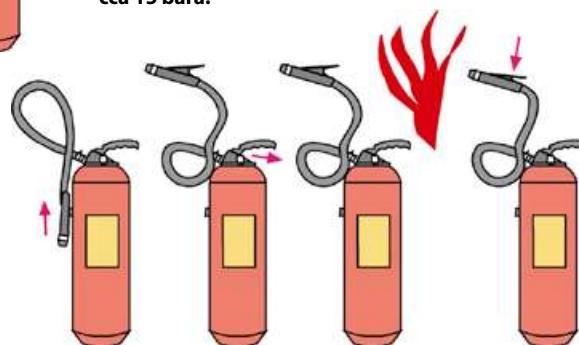
Sl. 56. Postupak aktiviranja aparata za početno gašenje požara: 1. donjeti aparat na prihvatljivu udaljenost od požara, uhvatiti mlaznicu, 2. izvući osigurač, 3. usmjeriti mlaznicu prema požaru, 4. pritisnuti ručicu na aparatu i ručicu na mlaznici na crijevu (ukoliko je izvedena)
